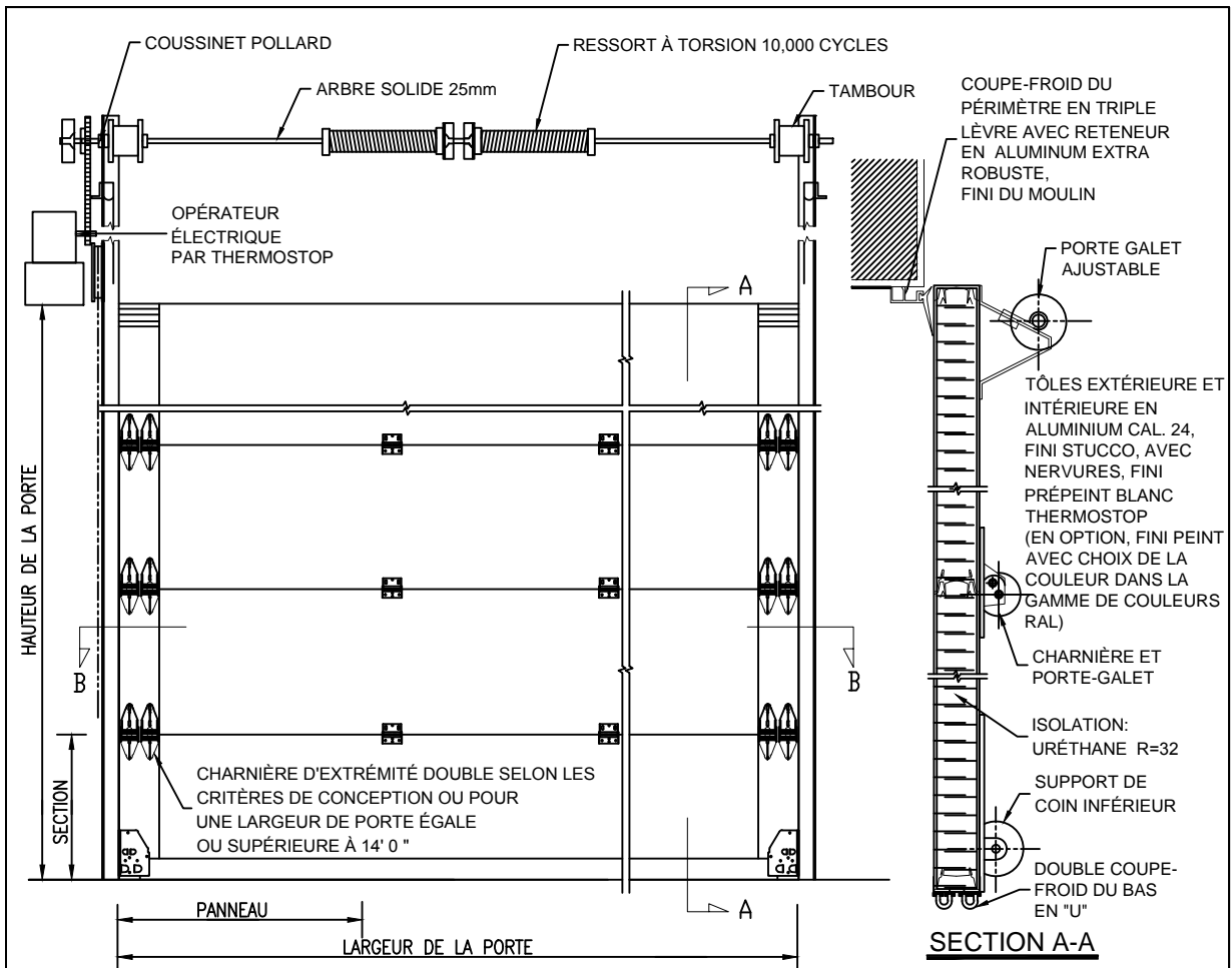
ÉLÉVATION INTÉRIEURE
