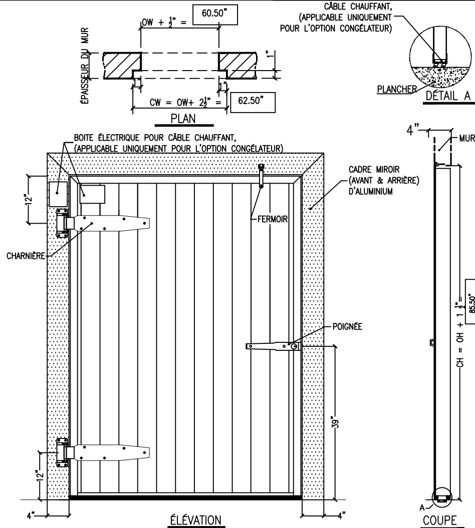
DÉTAIL DU CADRE MIROIR (AVANT & ARRIÈRE) DE PORTE
