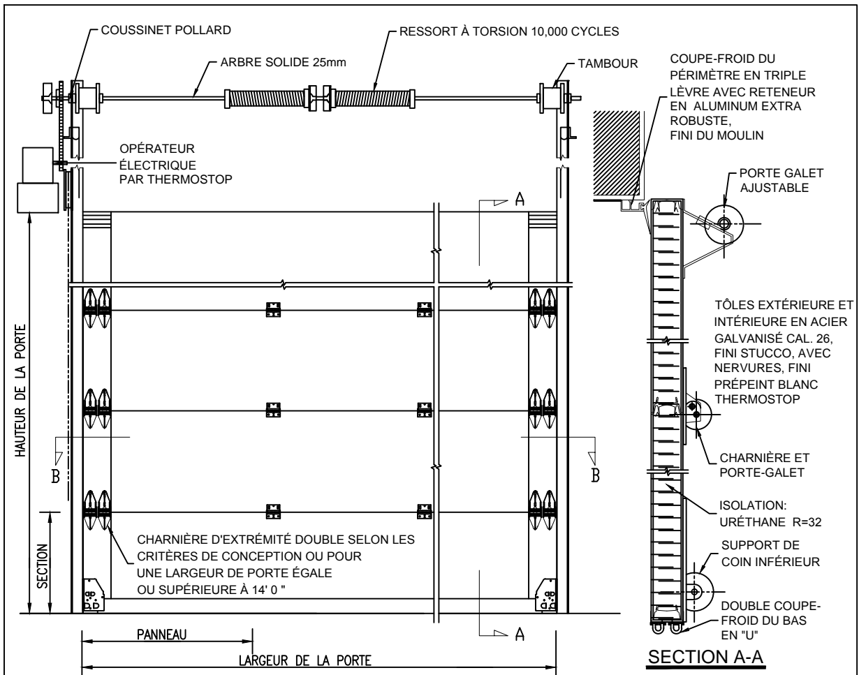
ÉLEVATION INTÉRIEURE
